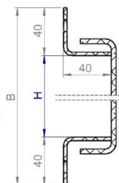
COUPE B-B
